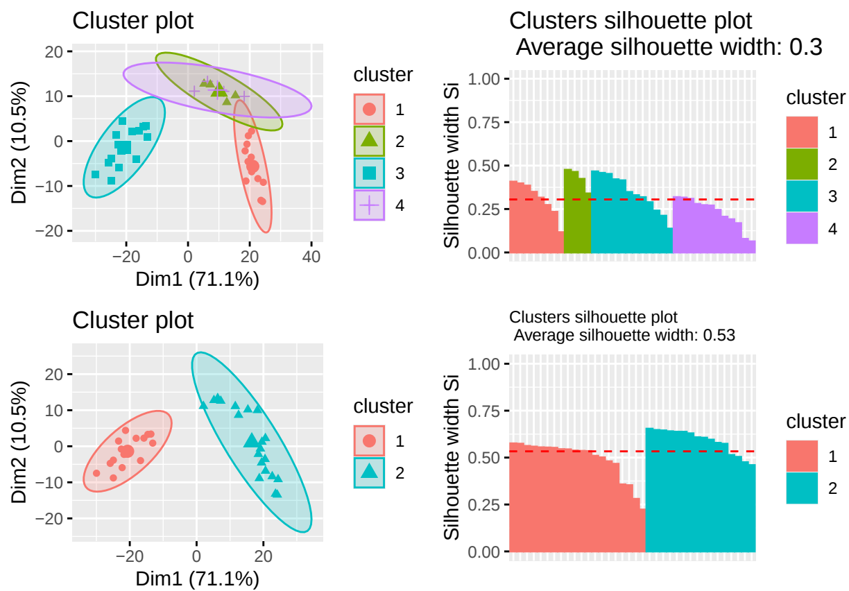
Figure 9: Visualisation des clusters générés par la méthode kmeans dans le plan factoriel 1,2
