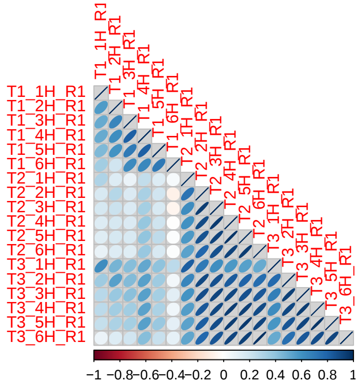
Figure 4: Visualisation de la matrice de covariance des variables quantitatives sur le réplicat R1
