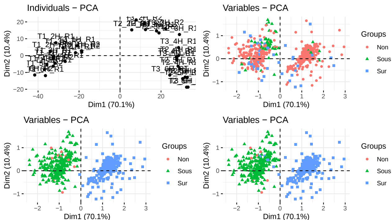
Figure 6: Projection des individus dans le plan factoriel et corrélations des variables avec les composantes principales
