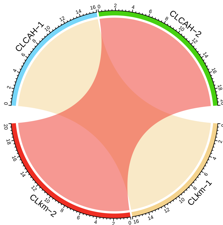
Figure 12: Diagramme mettant en valeur l'exacte correspondance des classes entre les deux clusterings
