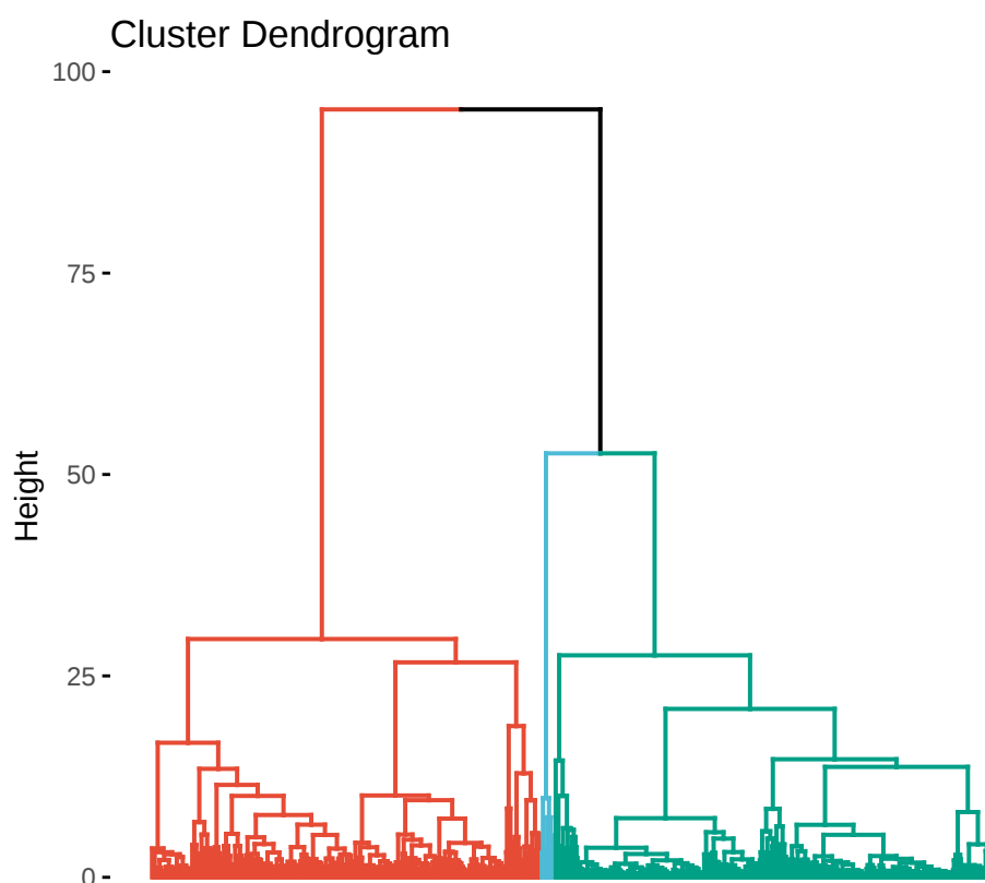
Figure 18: Dendrogramme du clustering de l'ACP, obtenu par méthode CAH
